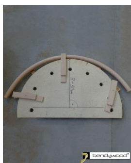
Ritorno elastico dopo aver tolto il pezzo dalla dima
