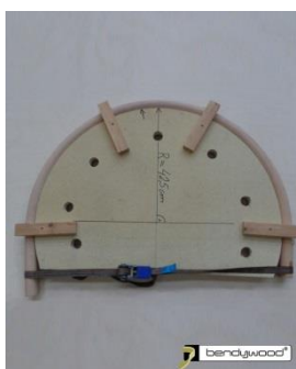
Esempio di una comune dima per piegare
